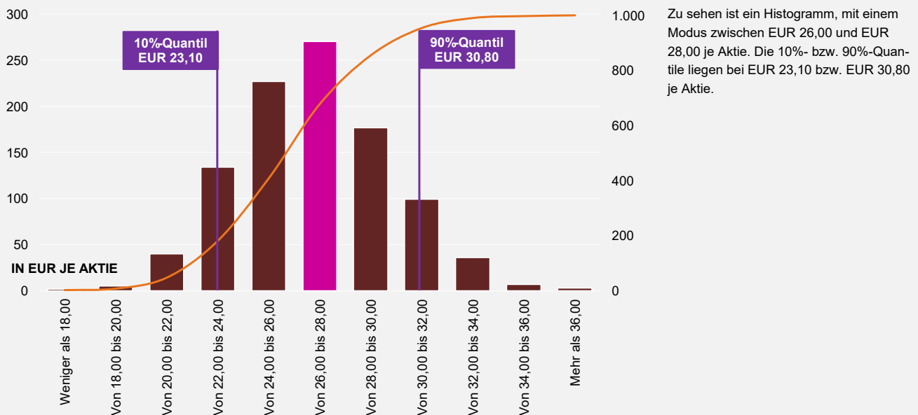
ABBILDUNG 1: MONTE CARLO-SIMULATION
